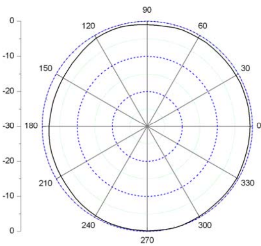
H-Plane
