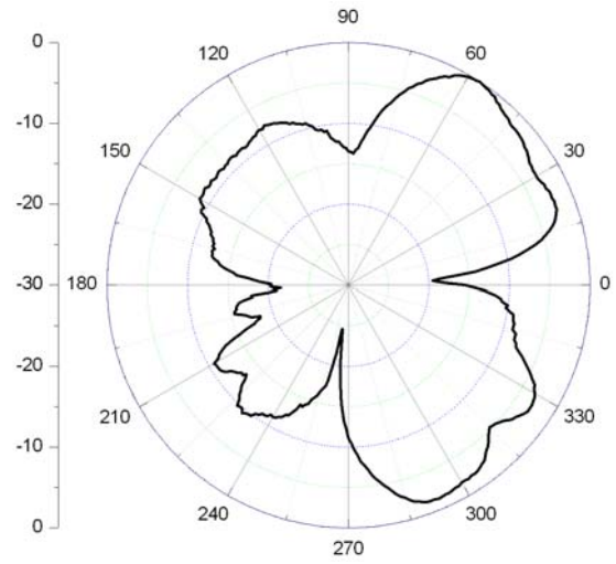
E-Plane
