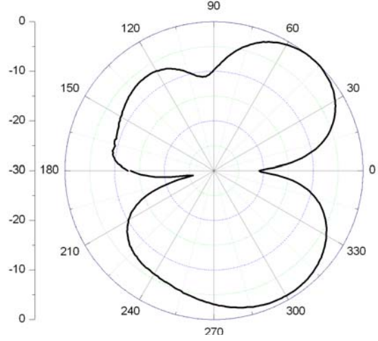
E-Plane
