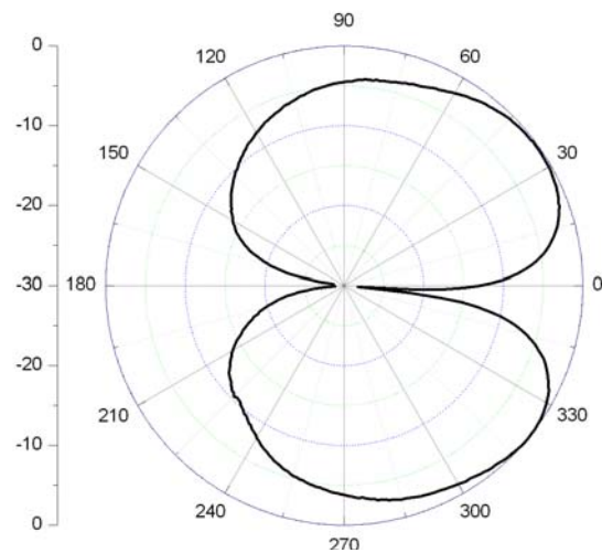
E-Plane
