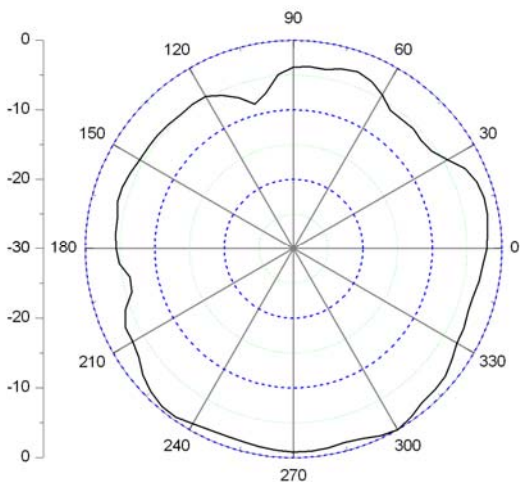
H-Plane
