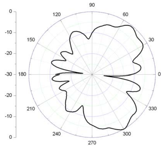
E-Plane
